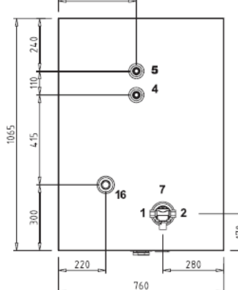
Top view CU 750
